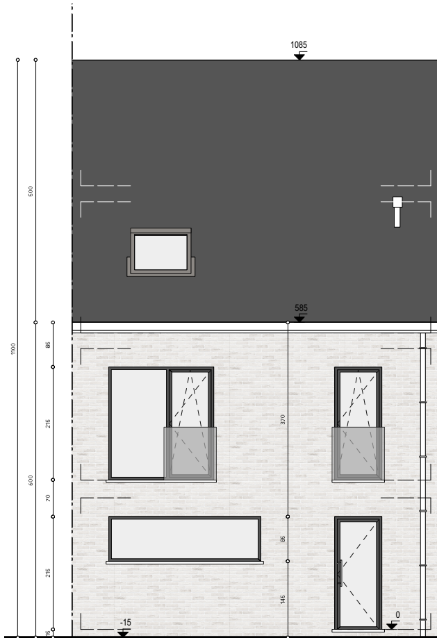
aanzicht voorgevel
