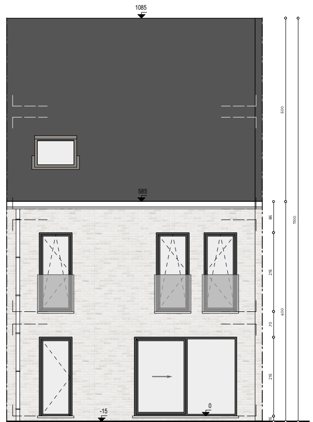
aanzicht achtergevel
