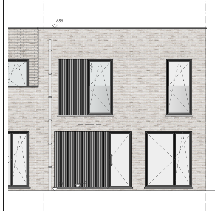
aanzicht voorgevel
