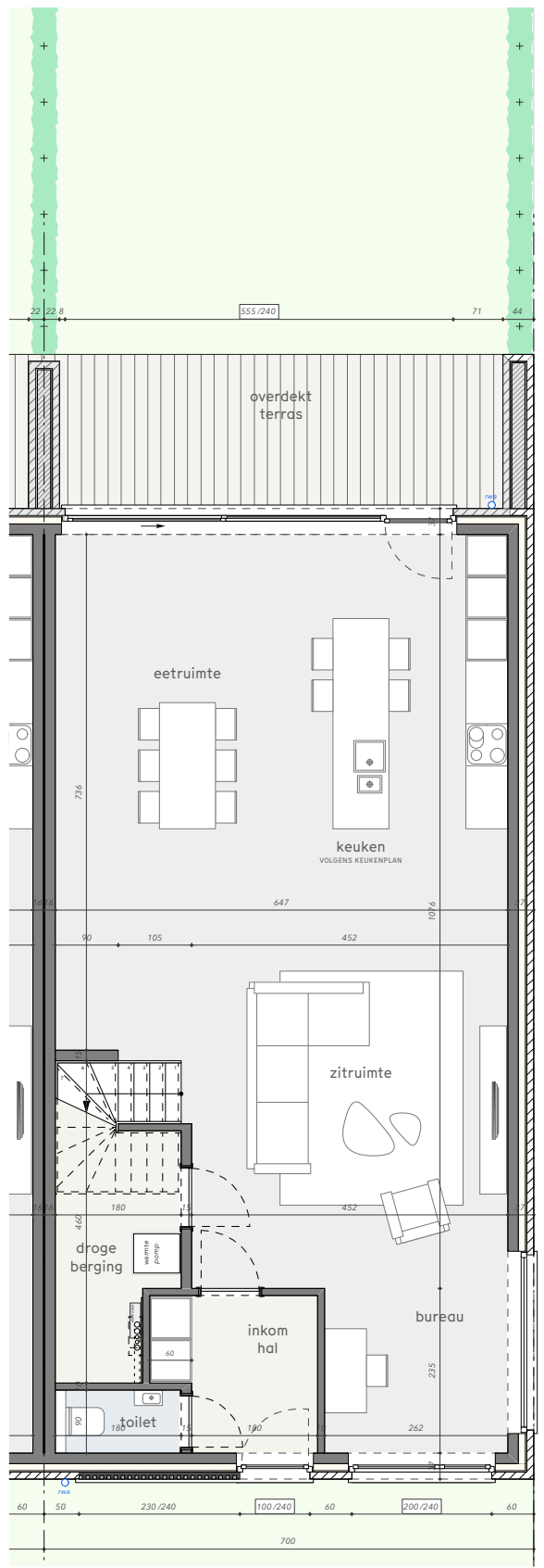
grondplan gelijkvloers
