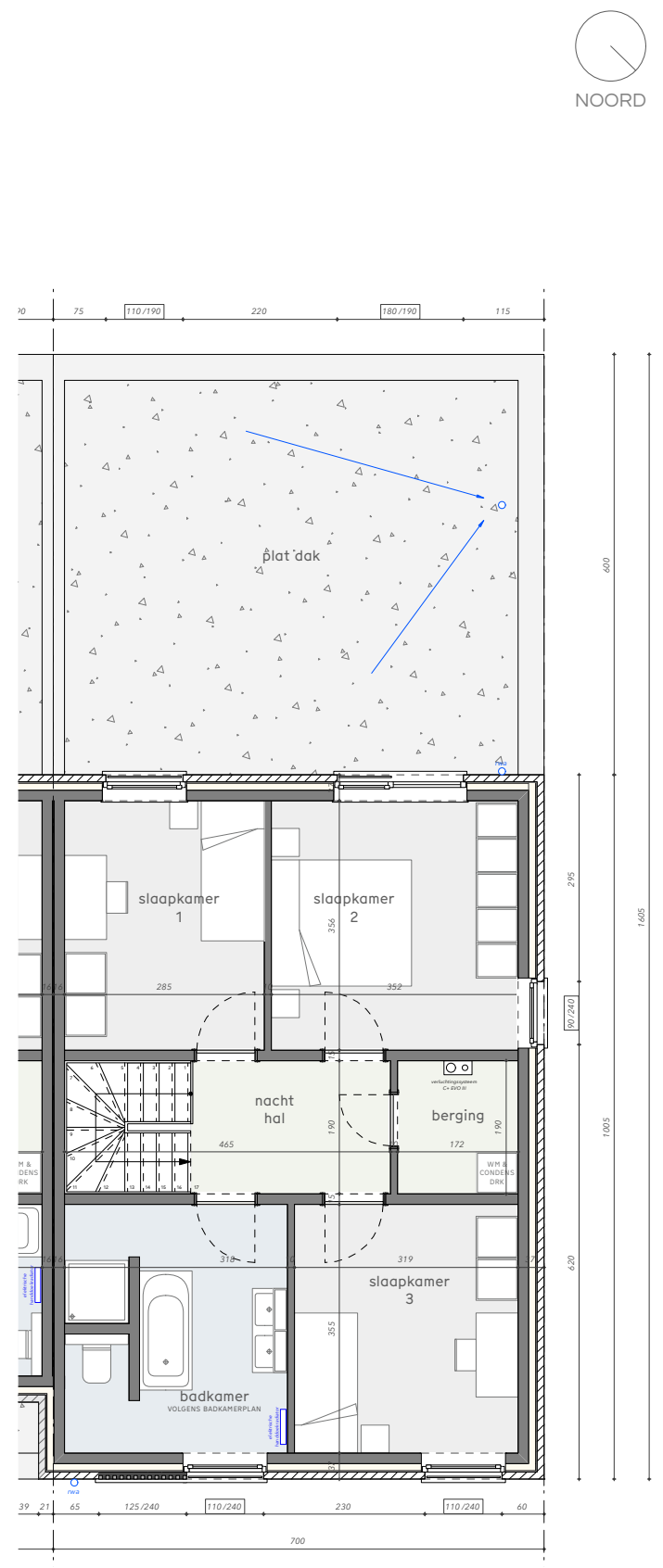
grondplan verdieping
