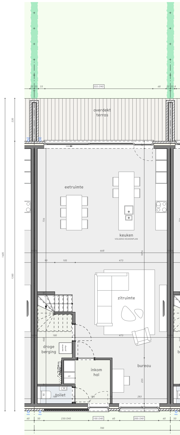
grondplan gelijkvloers
