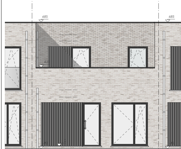
aanzicht voorgevel
