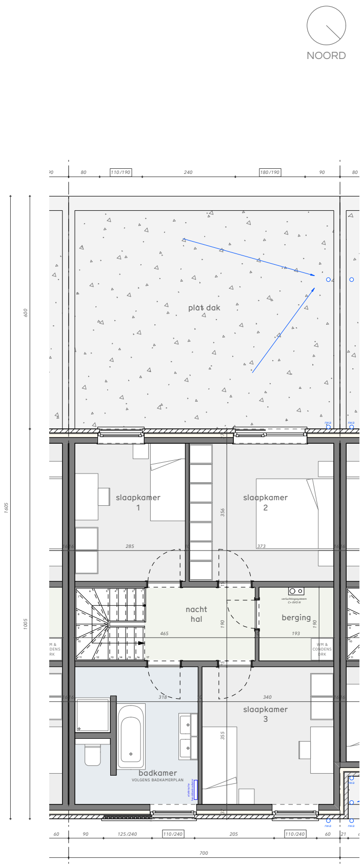
grondplan verdieping
