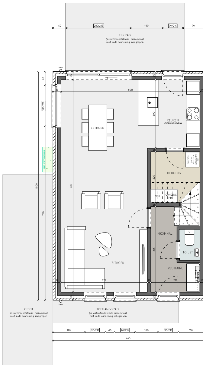
grondplan gelijkvloers
