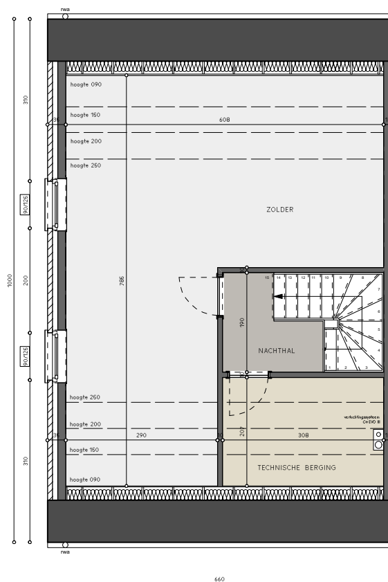
grondplan zolder
